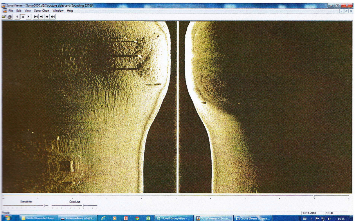
Nogmaals oude betonpalen met de harde schaduw aan de achterzijde. De schaduw wordt veroorzaakt doordat de StructureScan niet achter de palen kan kijken.
